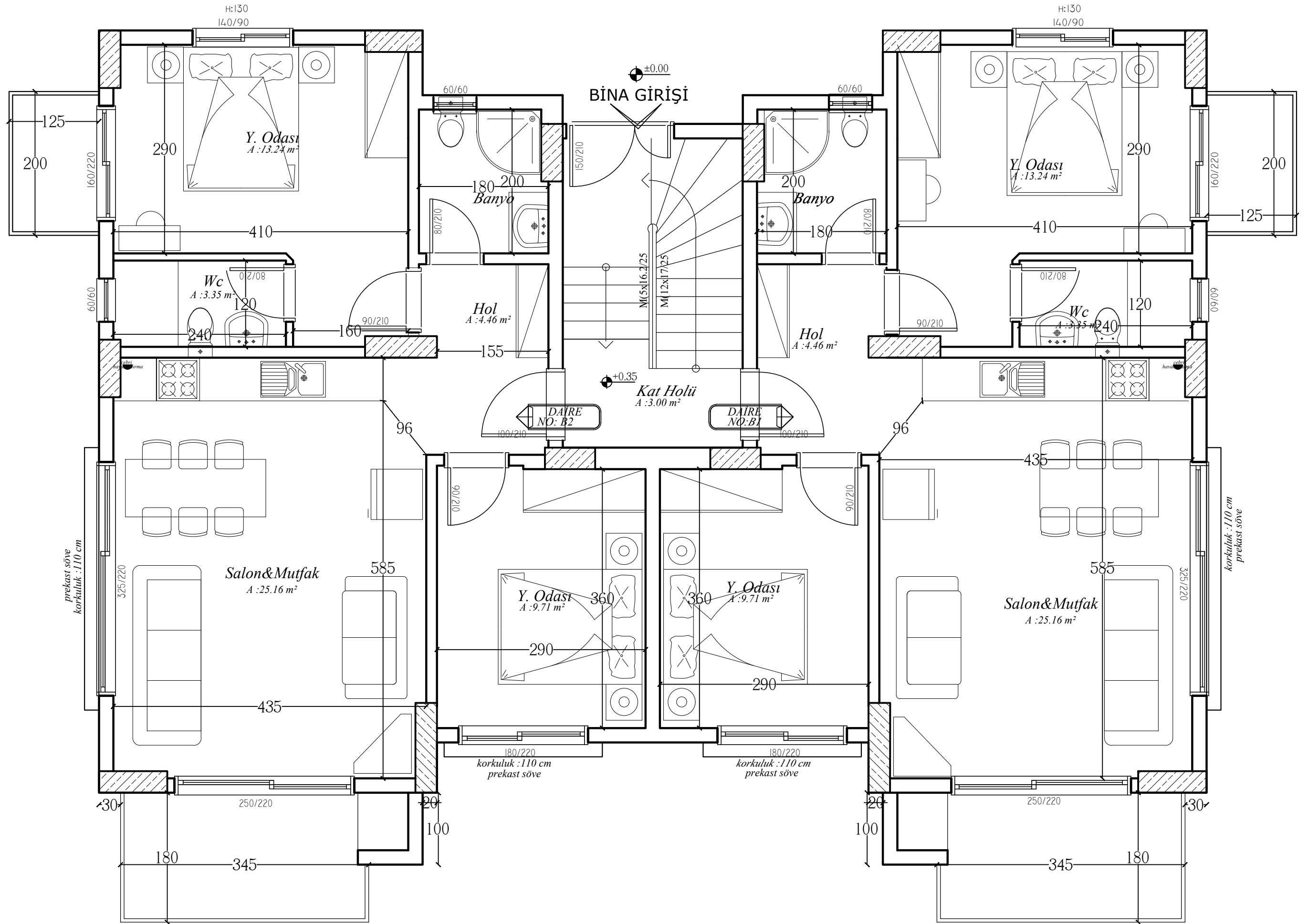
B BLOK Zemin kat Planı
