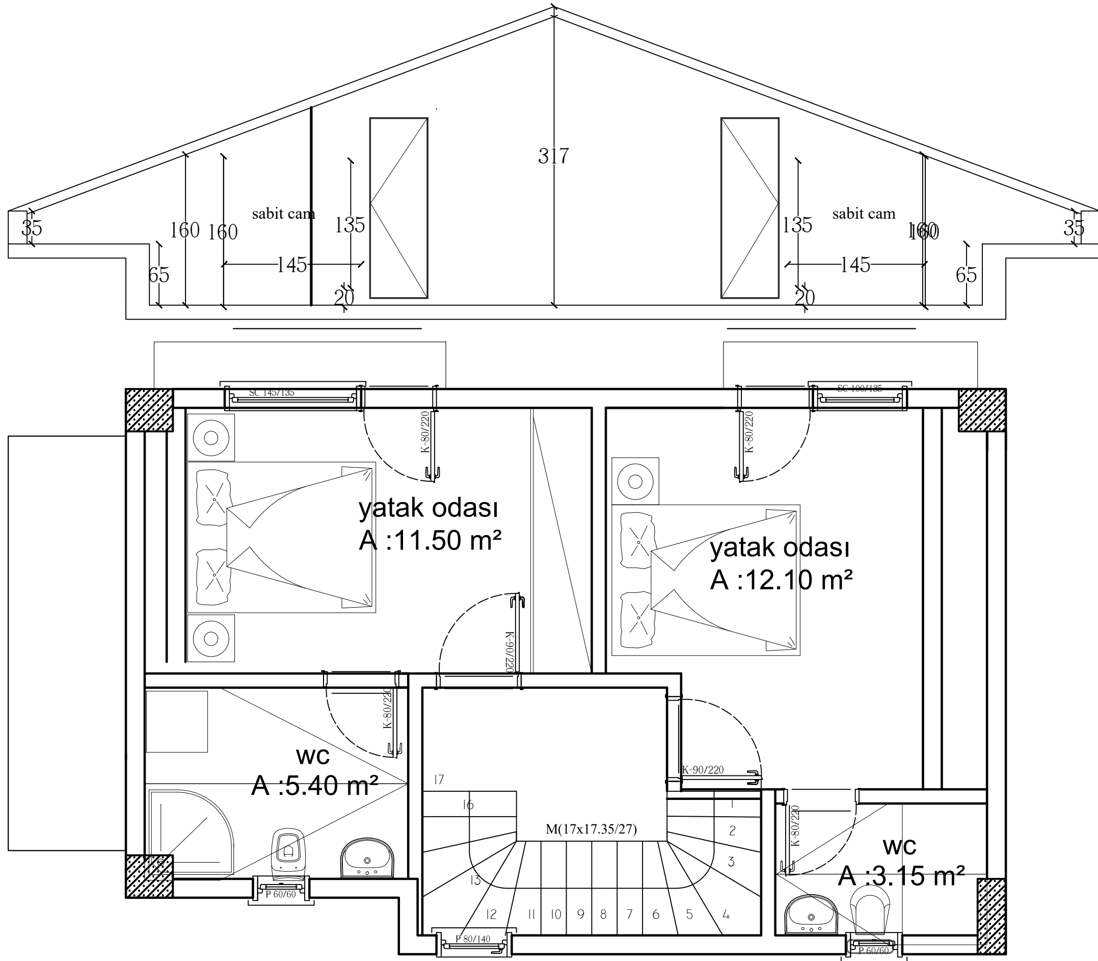
Çatı Kat Planı
